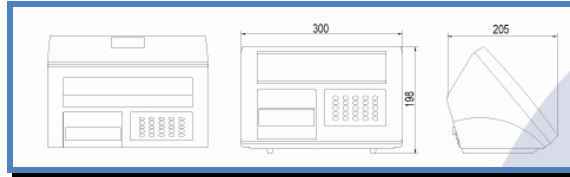
Dimensiones externas
